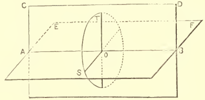
Fig. 3.—Dihedral Angles.
